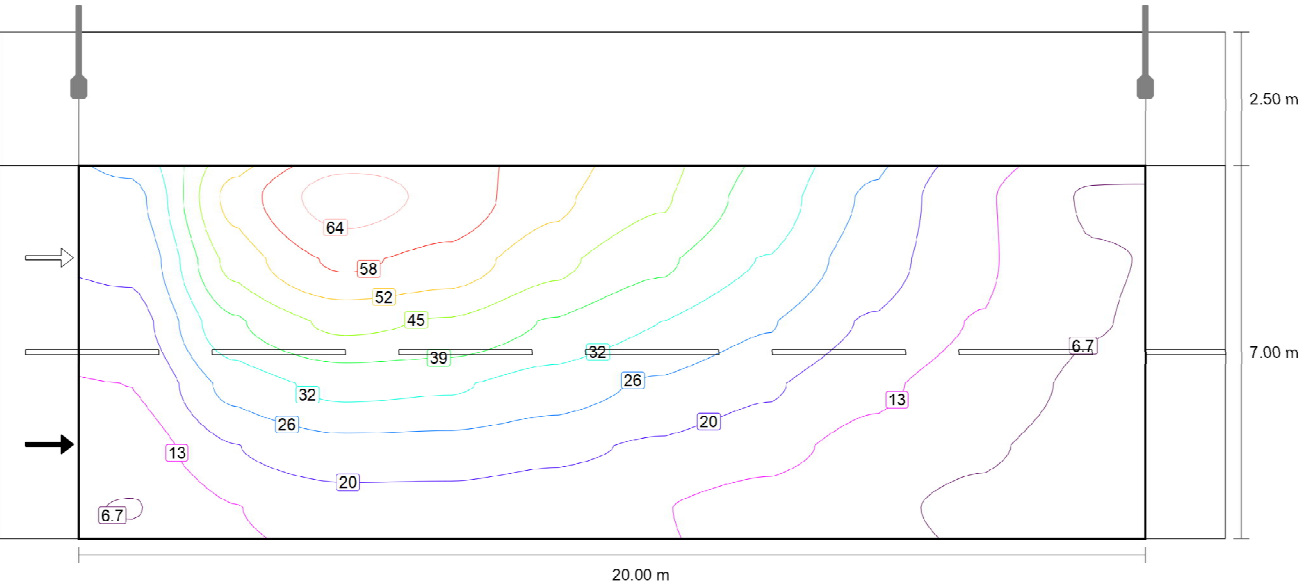
Valor de manutenção de iluminância vertical (oeste) [lx] (Linhas de isolux)
