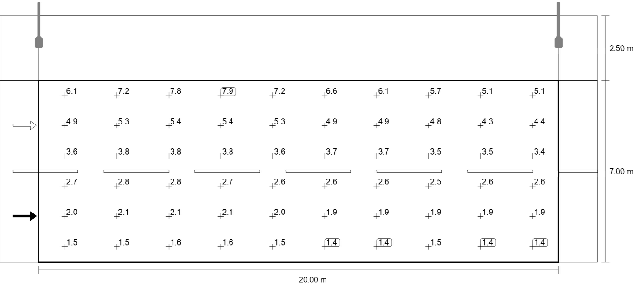
Observador 1: Luminância com instalação nova [cd/m²] (Grelha de valores)
