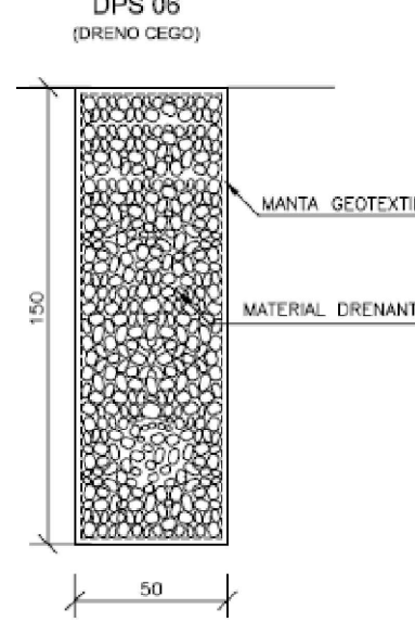
Detalhe Escavação de Bueiros DETALHE DA ESCAVAÇÃO DE VALAS PARA COLOCAÇÃO DE BUEIROS
