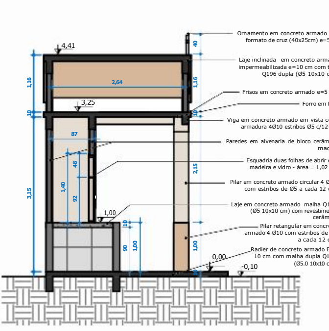
Corte B estrutural ESC: 1 : 50
