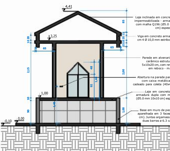
Corte A estrutural ESC: 1 : 50
